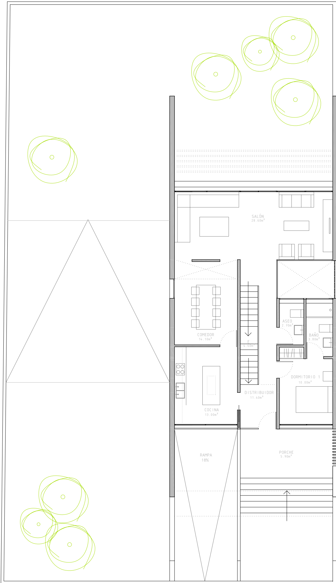
PLANTA BAJA
