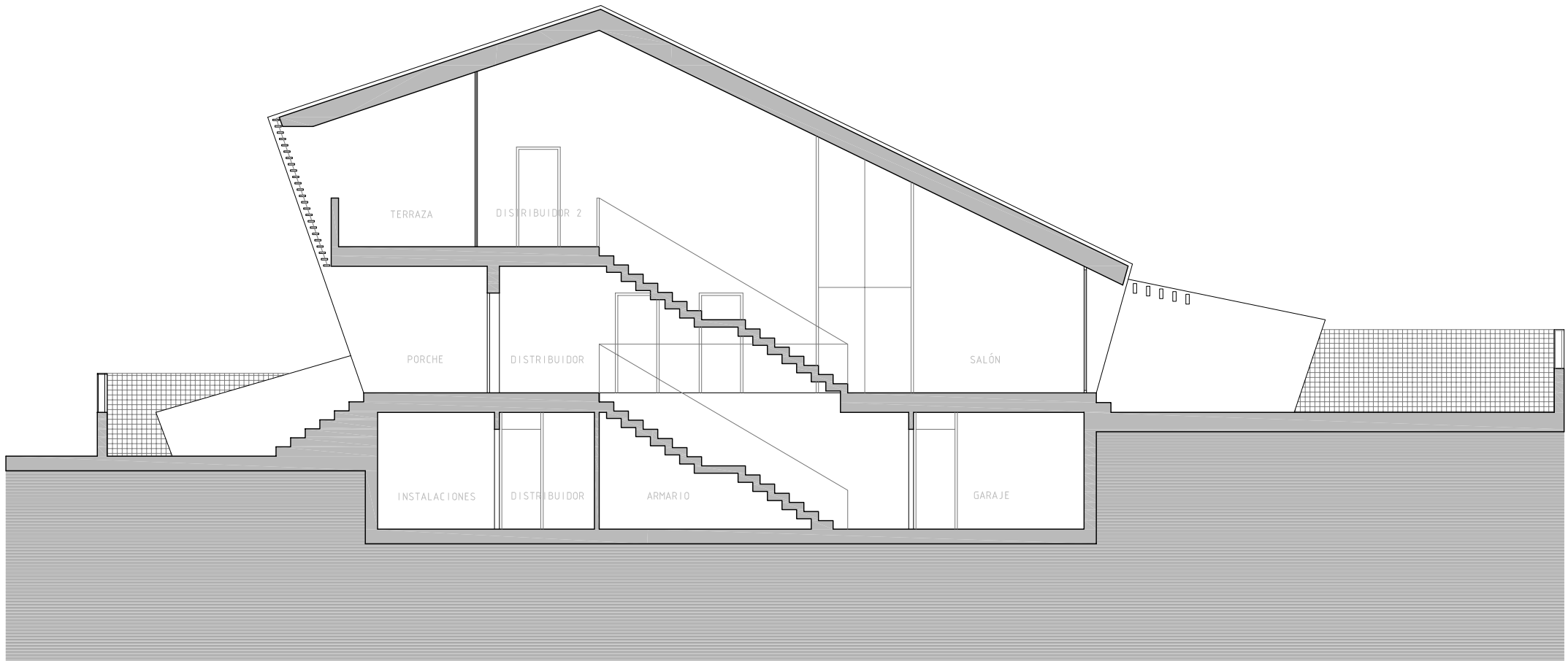
SECCIÓN ESCALERAS
