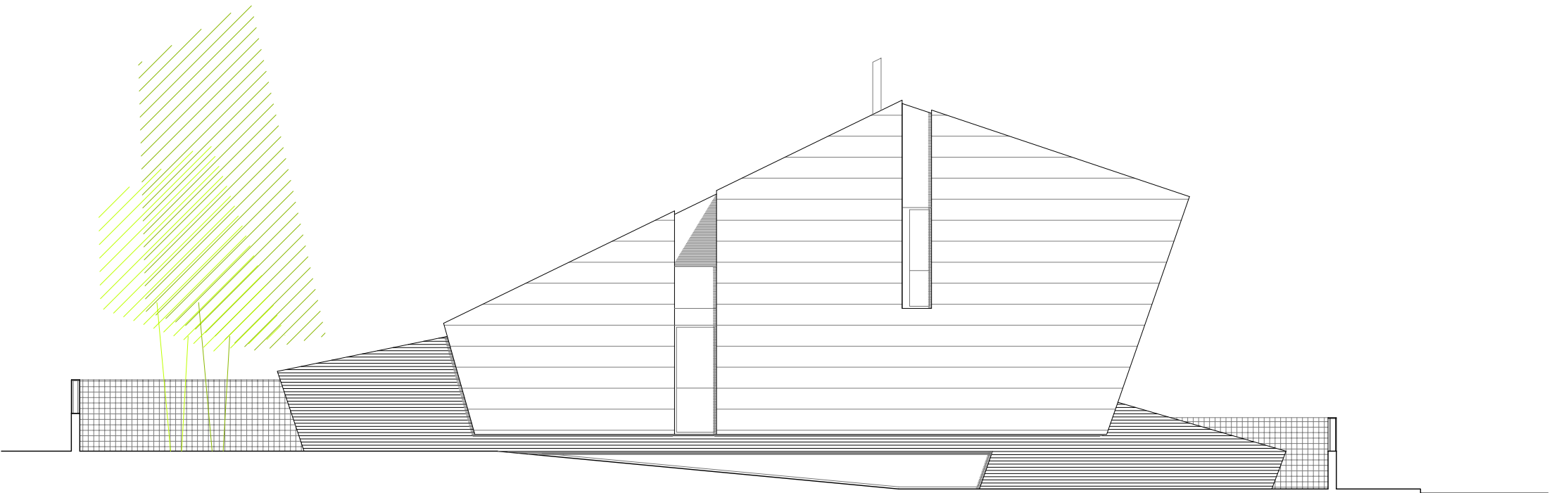
ALZADO LATERAL
