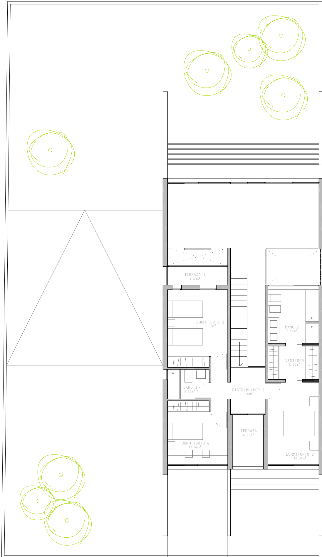
PLANTA PRIMERA
